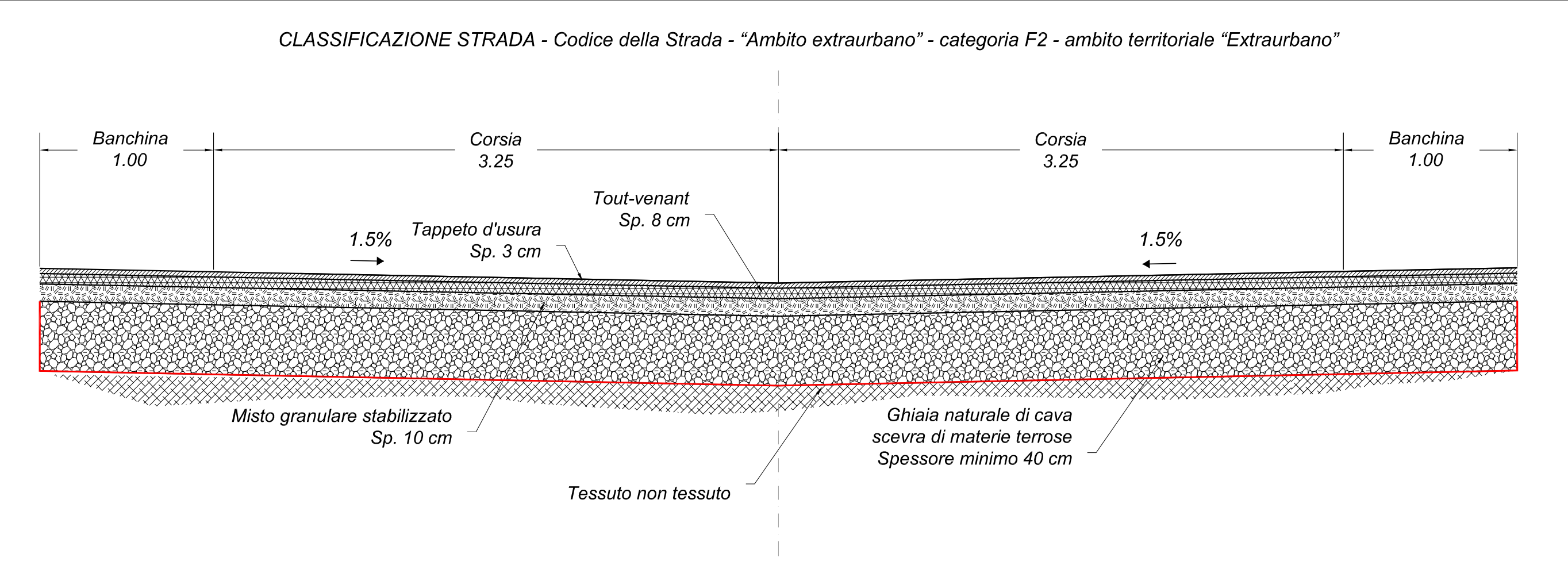
Sezione stradale tipo Scala 1:20
